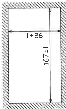
取付穴寸法図 (参考図) CUTOUT DIMENSIONS
