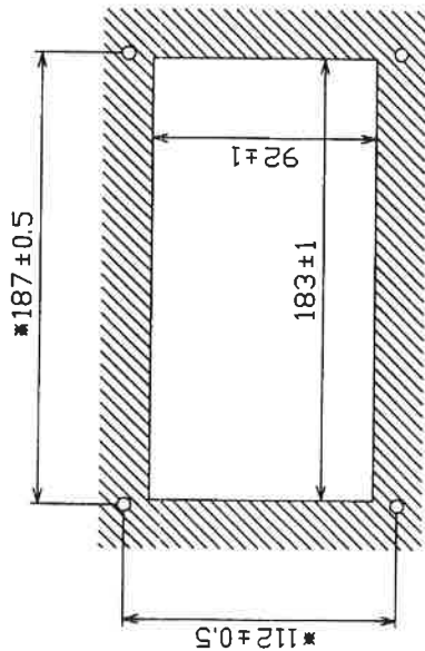
取付穴寸法図 (参考図) CUTOUT DIMENSIONS
