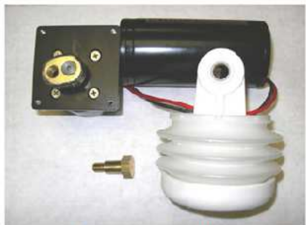
Kit con Motor Completo W y bellows
